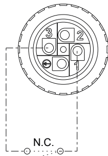
Fig. 11: Conexión de la protección ante funcionamiento en seco externa
