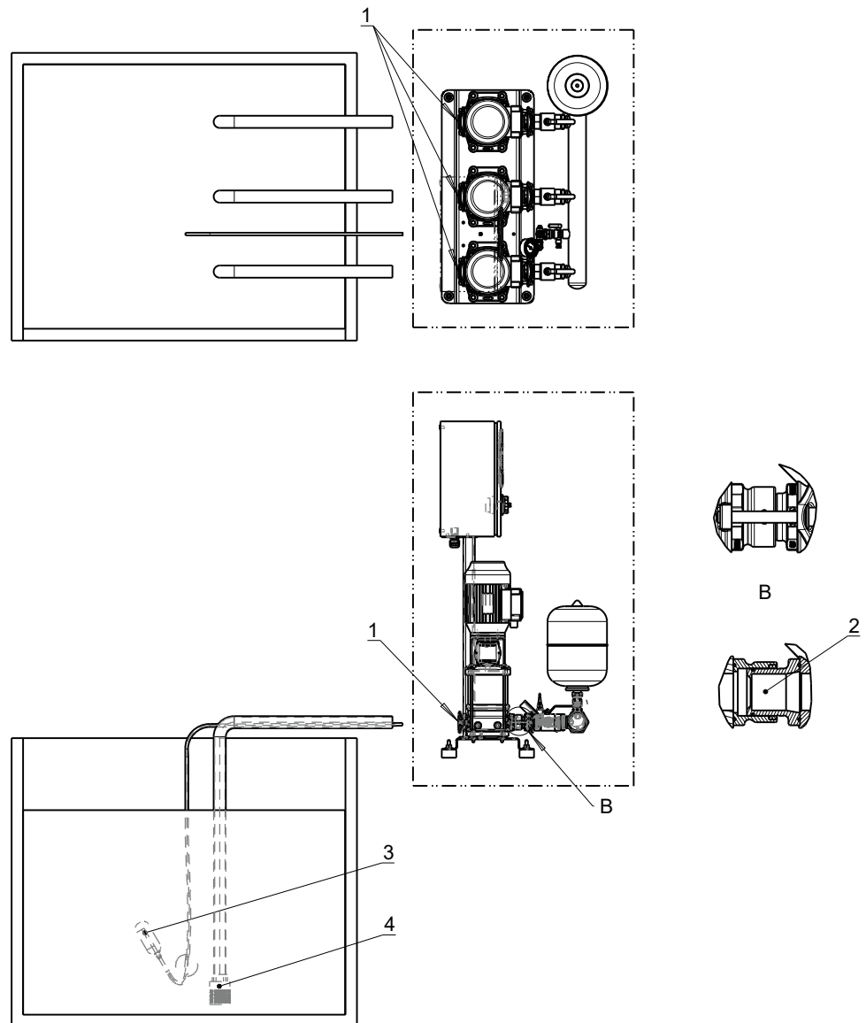
Fig. 8: Volumen de suministro del modelo L
