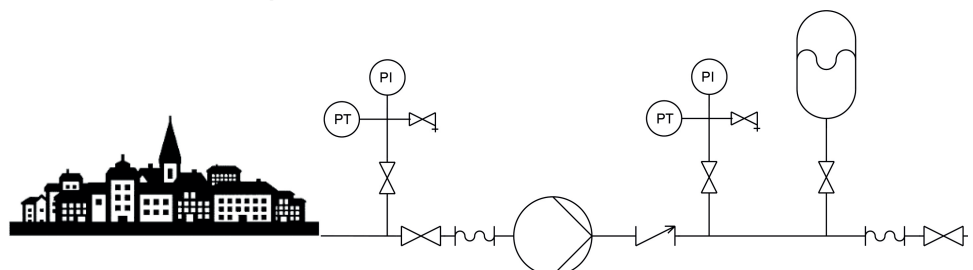
Fig. 3: M = la instalación de aumento de presión está conectada por el lado de aspiración al suministro de agua municipal, servicio en carga
