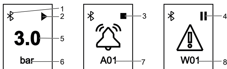
Fig. 13: Pantalla del convertidor de frecuencia, vista inicial
