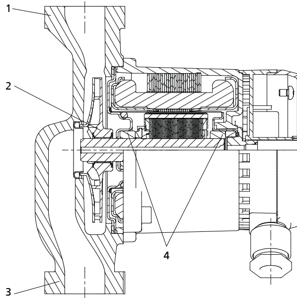
Fig. 2: Representación del grupo motobomba
