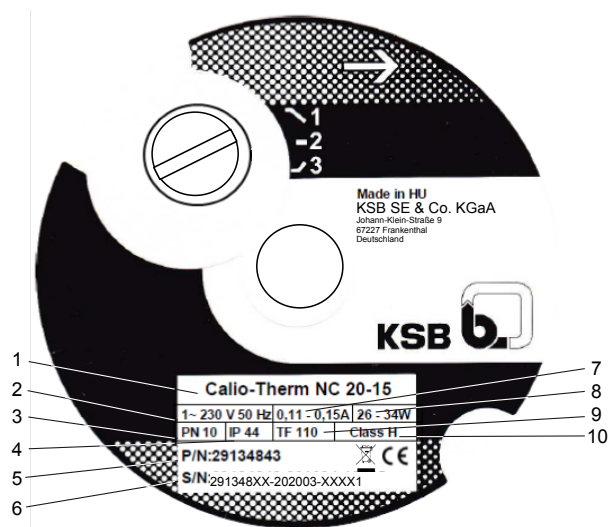
Fig. 1: Placa de características (ejemplo)
