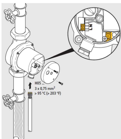
Fig. 4: Conexión del cableado eléctrico
