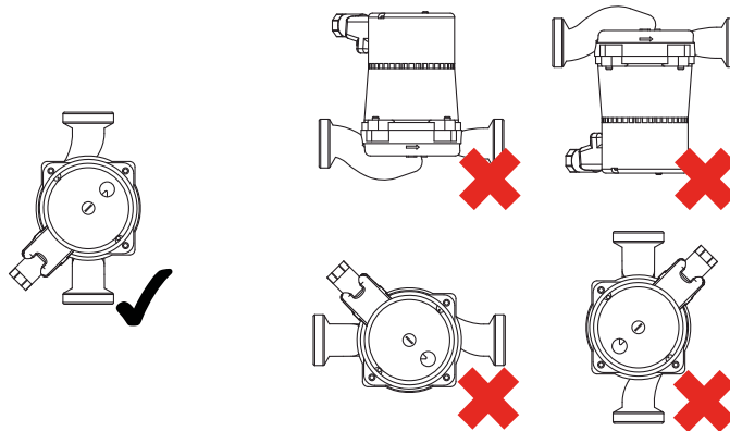
Fig. 3: Posiciones de montaje permitidas
