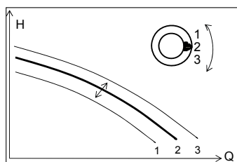
Fig. 6: Ajuste del modo de accionador
